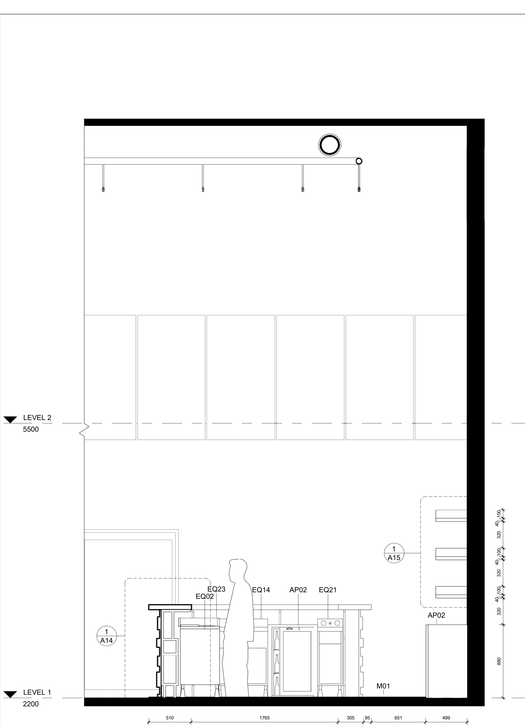
1 BAR Section 1 : 20
