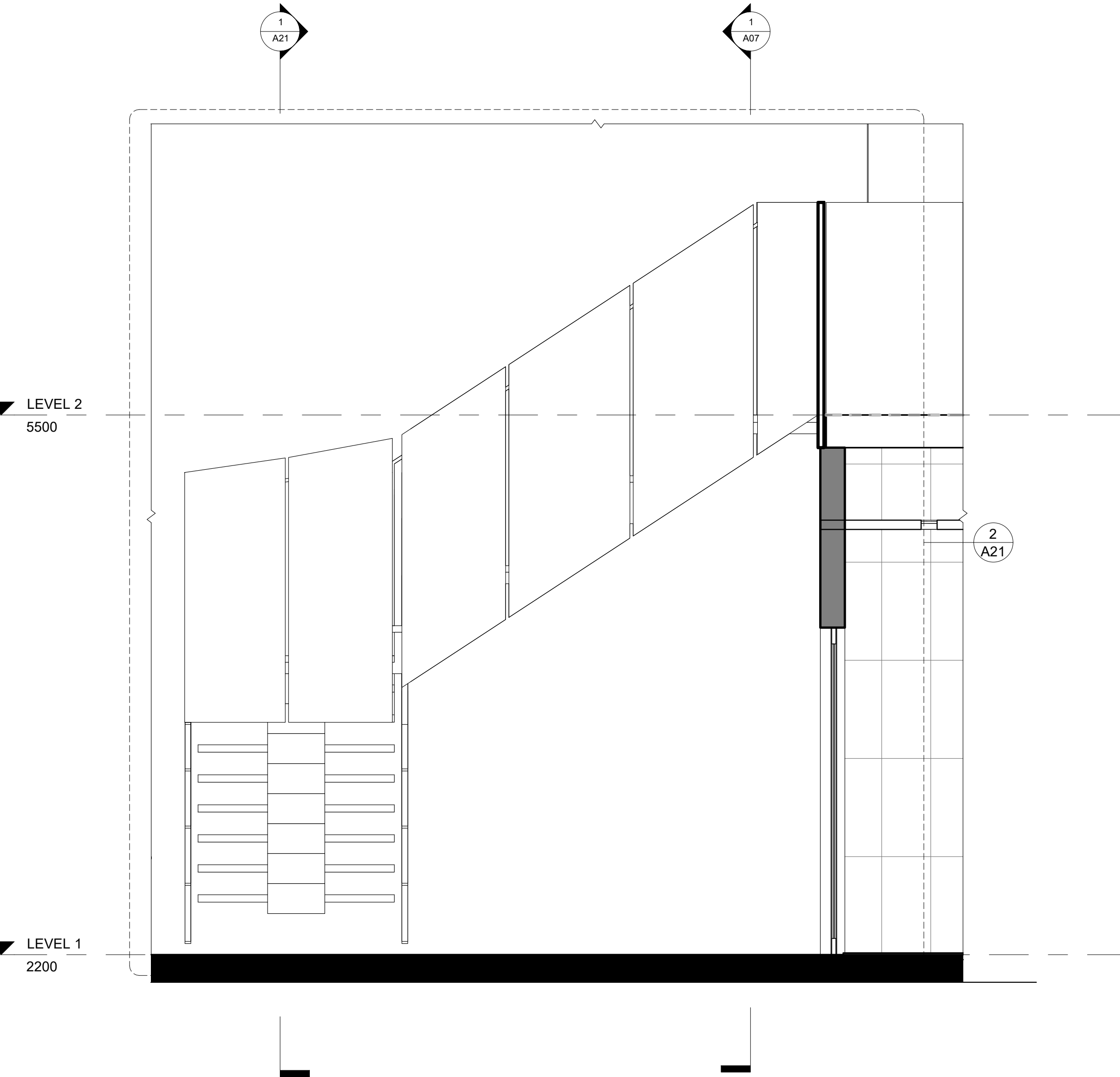
1 STAIR Elevation 3 1 : 20
