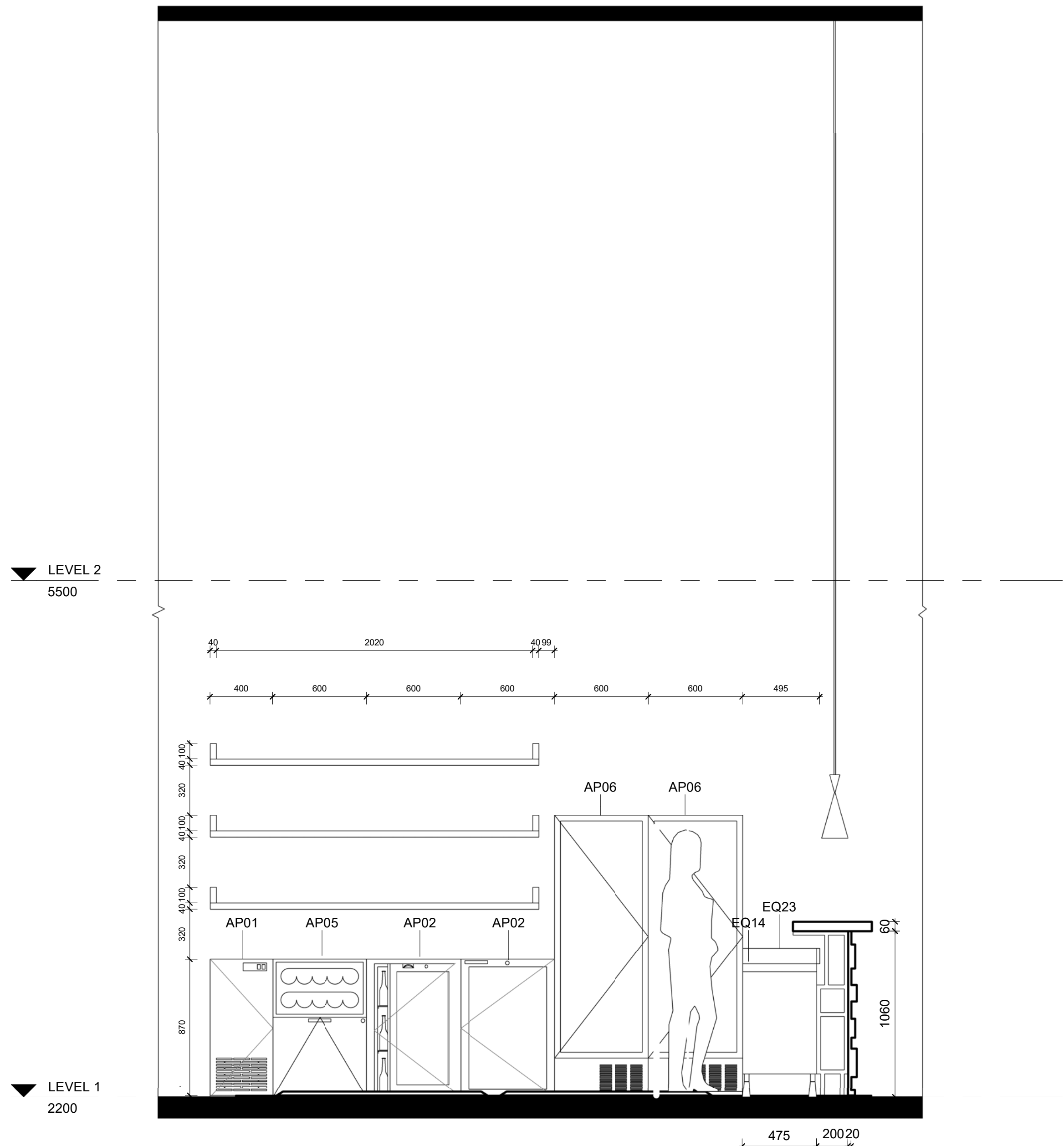
2 BAR Elevation 3 1 : 20
