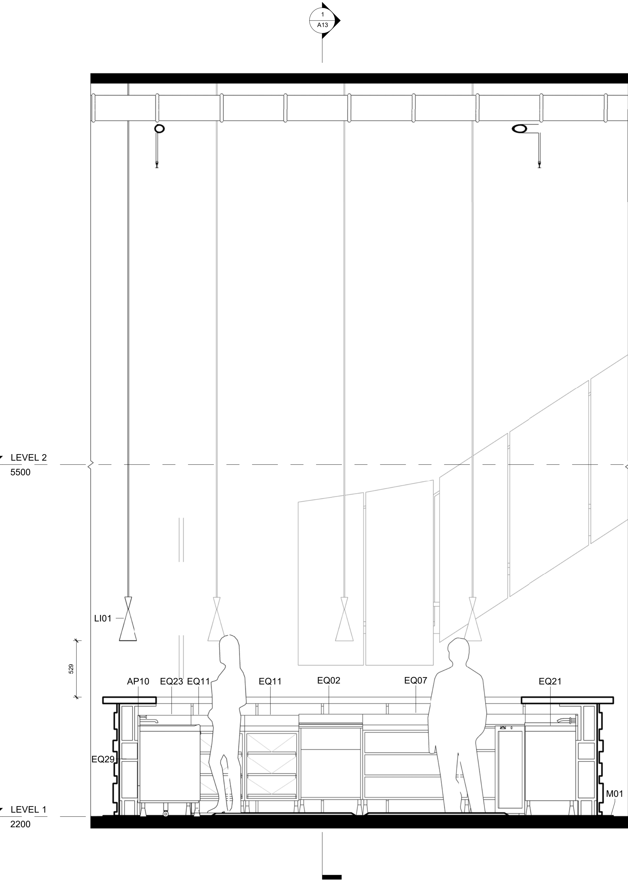
1 BAR Elevation 4 1 : 20
