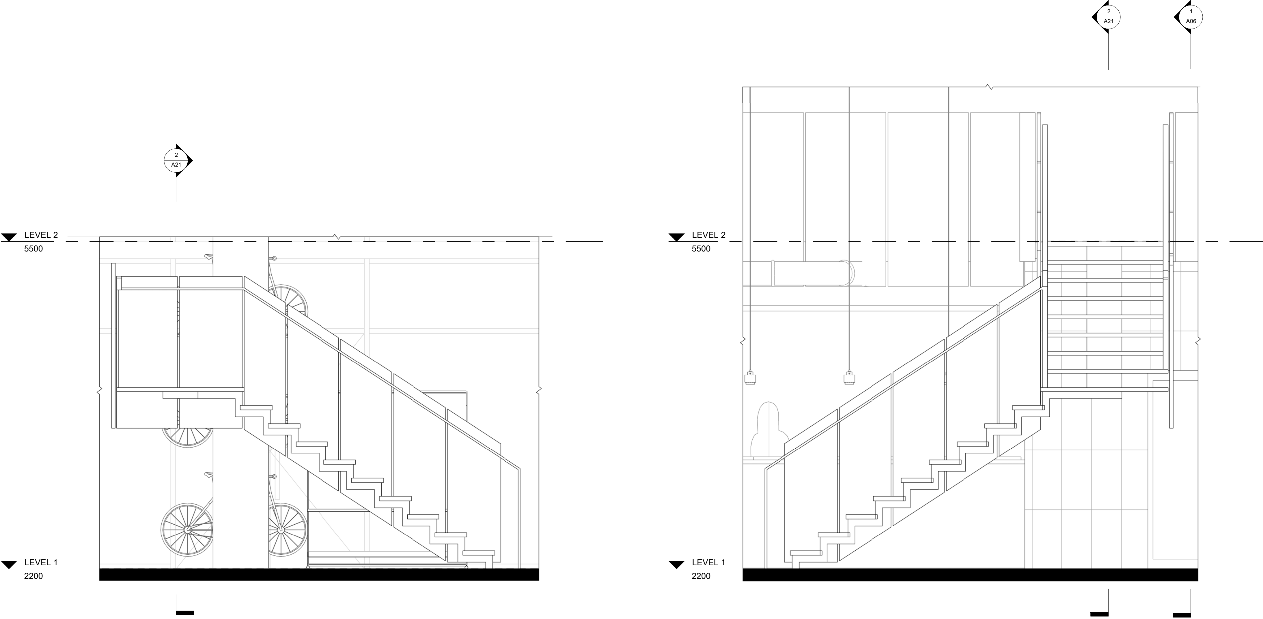
1 STAIR Elevation 5 1 : 20 2 STAIR Elevation 6 1 : 20
