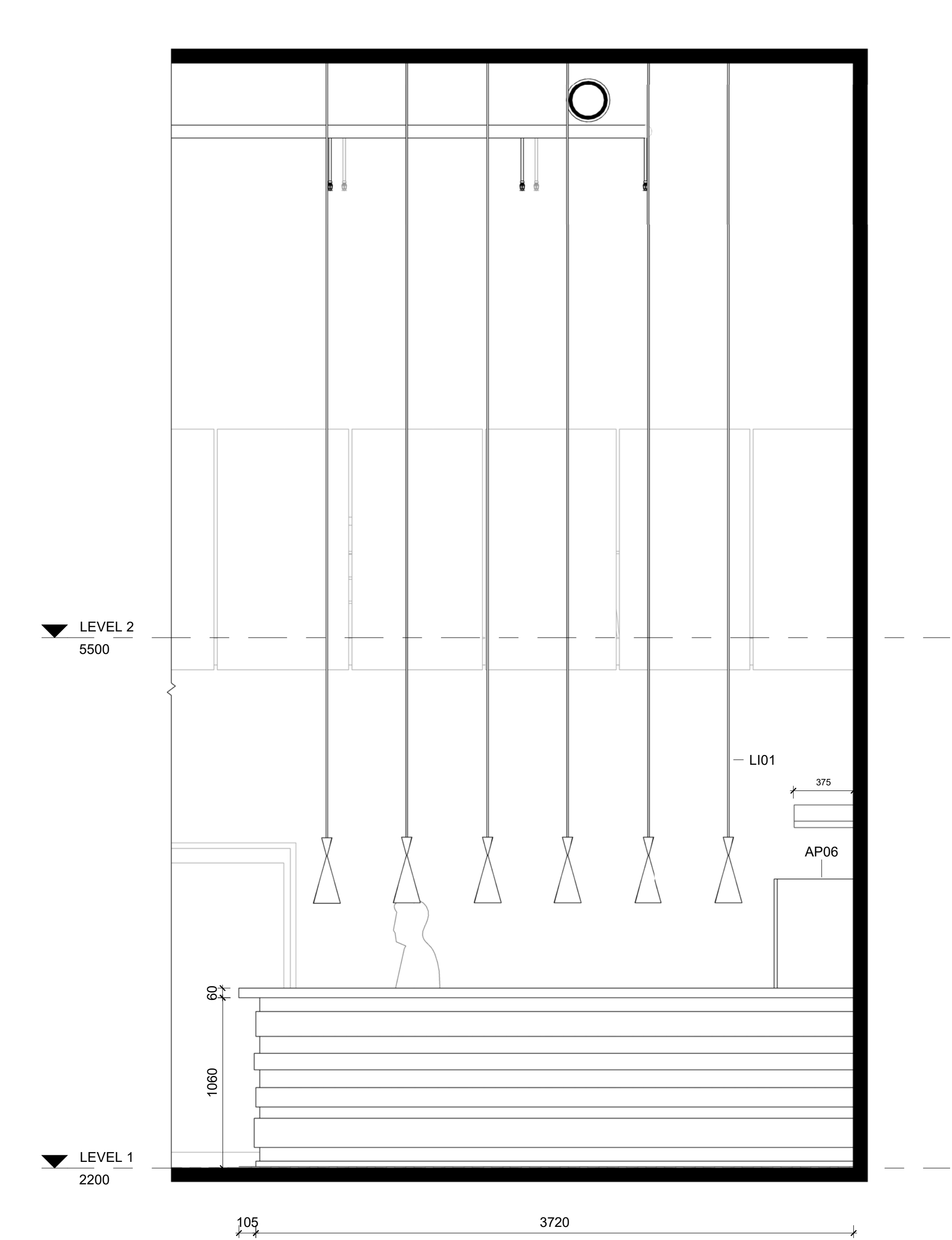
2 BAR Elevation 7 1 : 20
