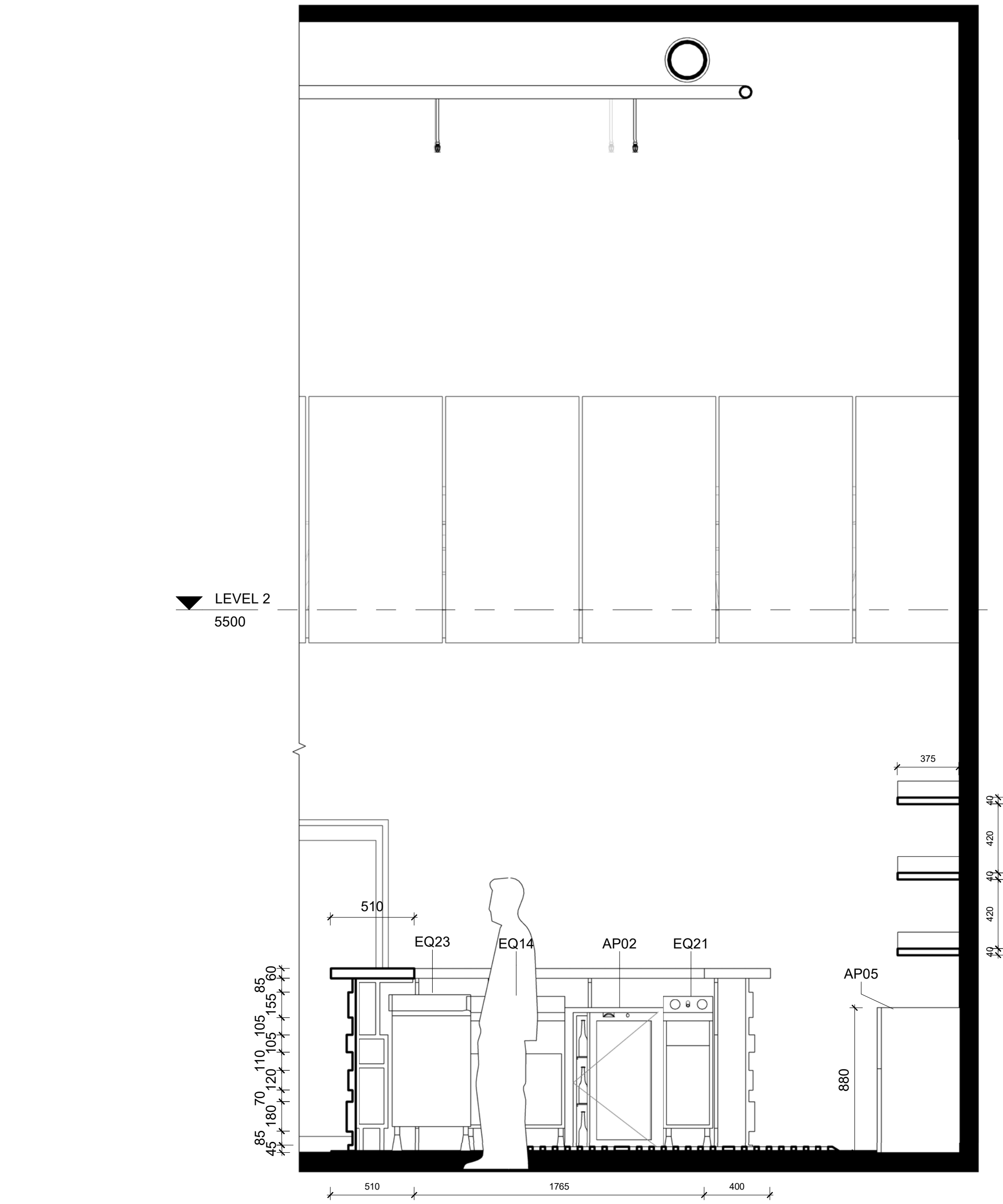
1 BAR Elevation 2 1 : 20
