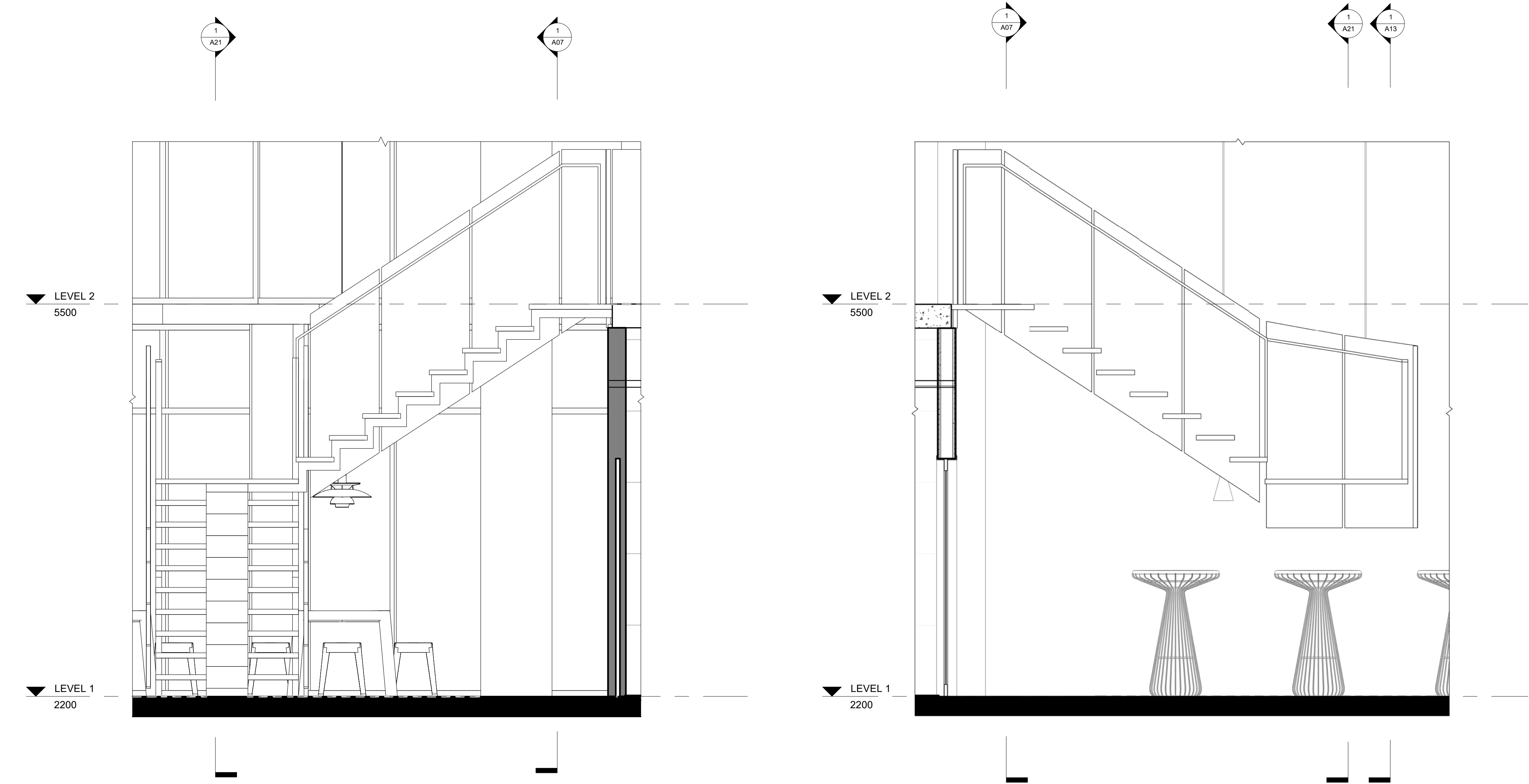
1 STAIR Elevation 7 1 : 20
