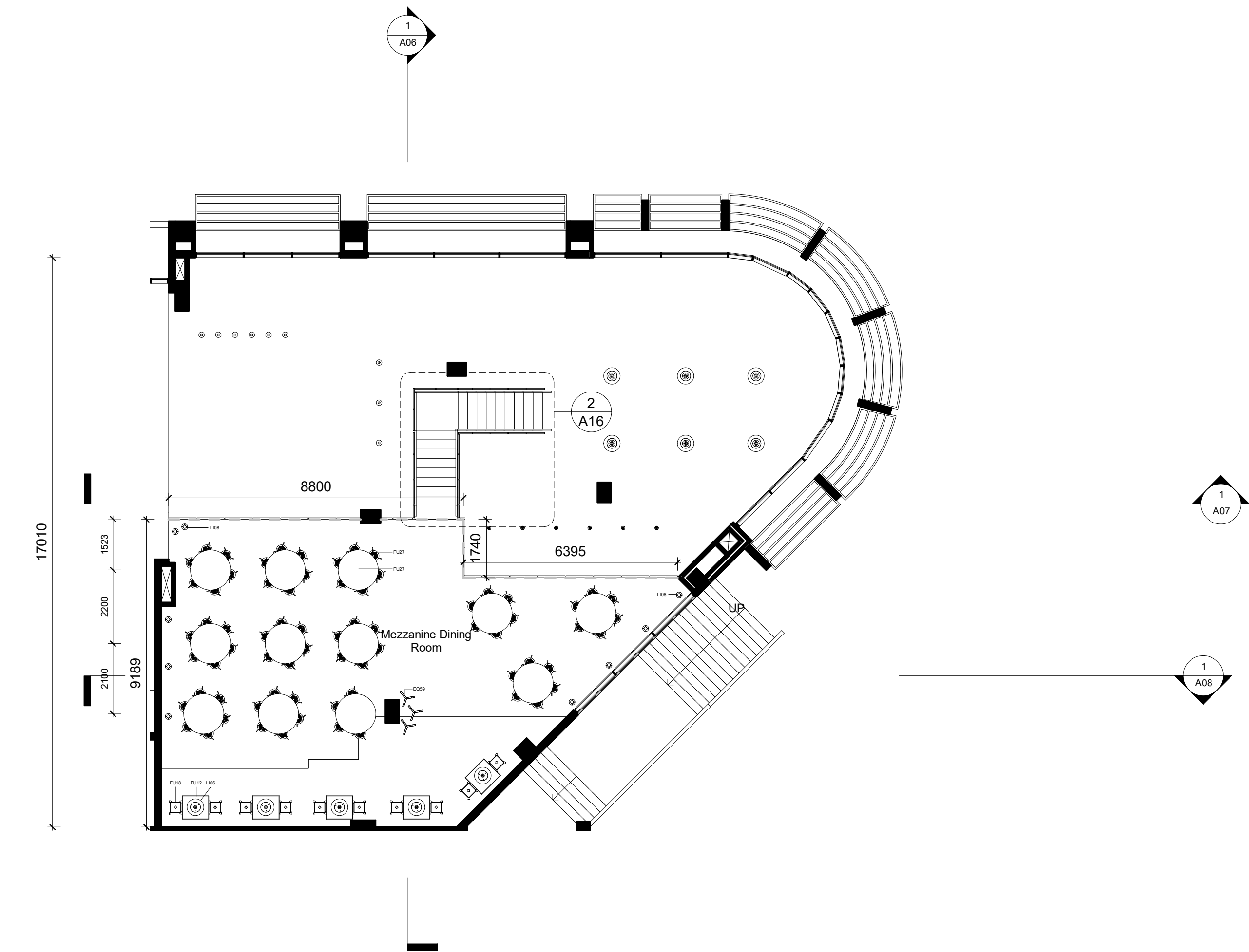
1 LEVEL 2 1 : 100
