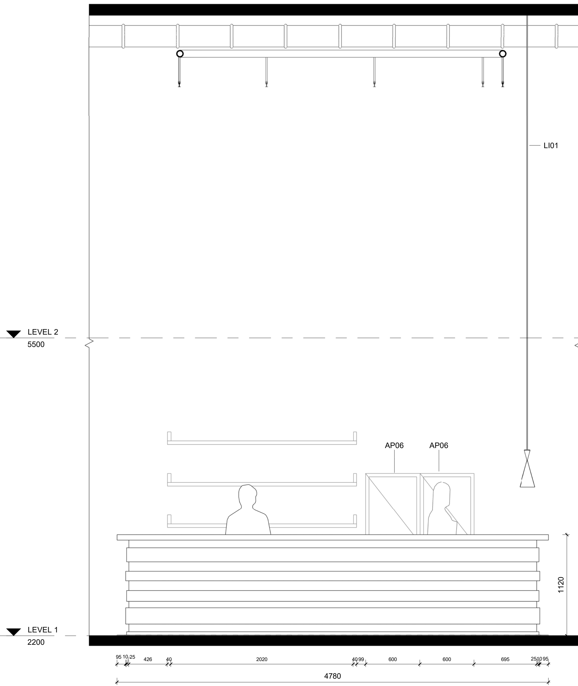
2 BAR Elevation 5 1 : 20
