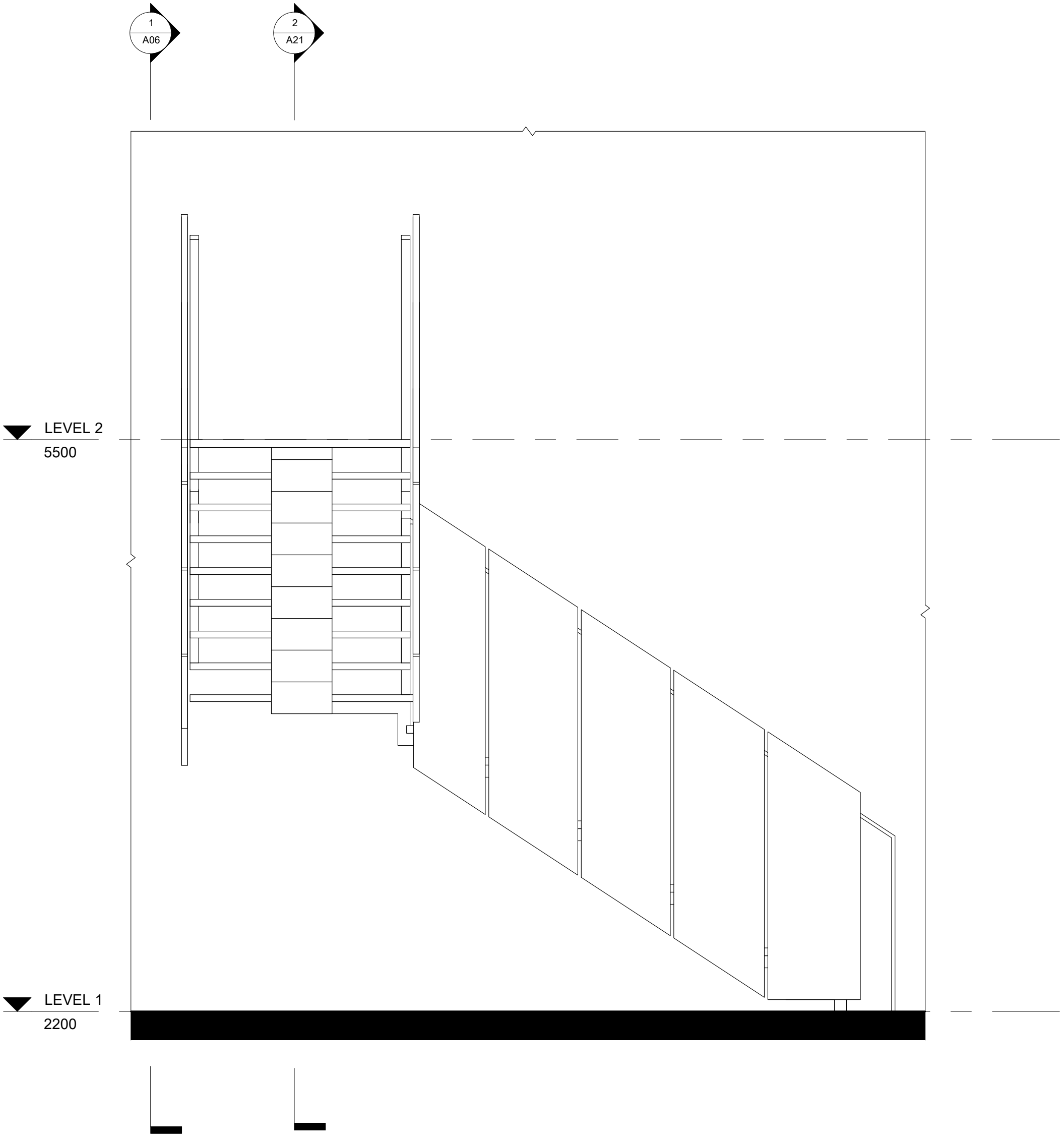
2 STAIR Elevation 4 1 : 20
