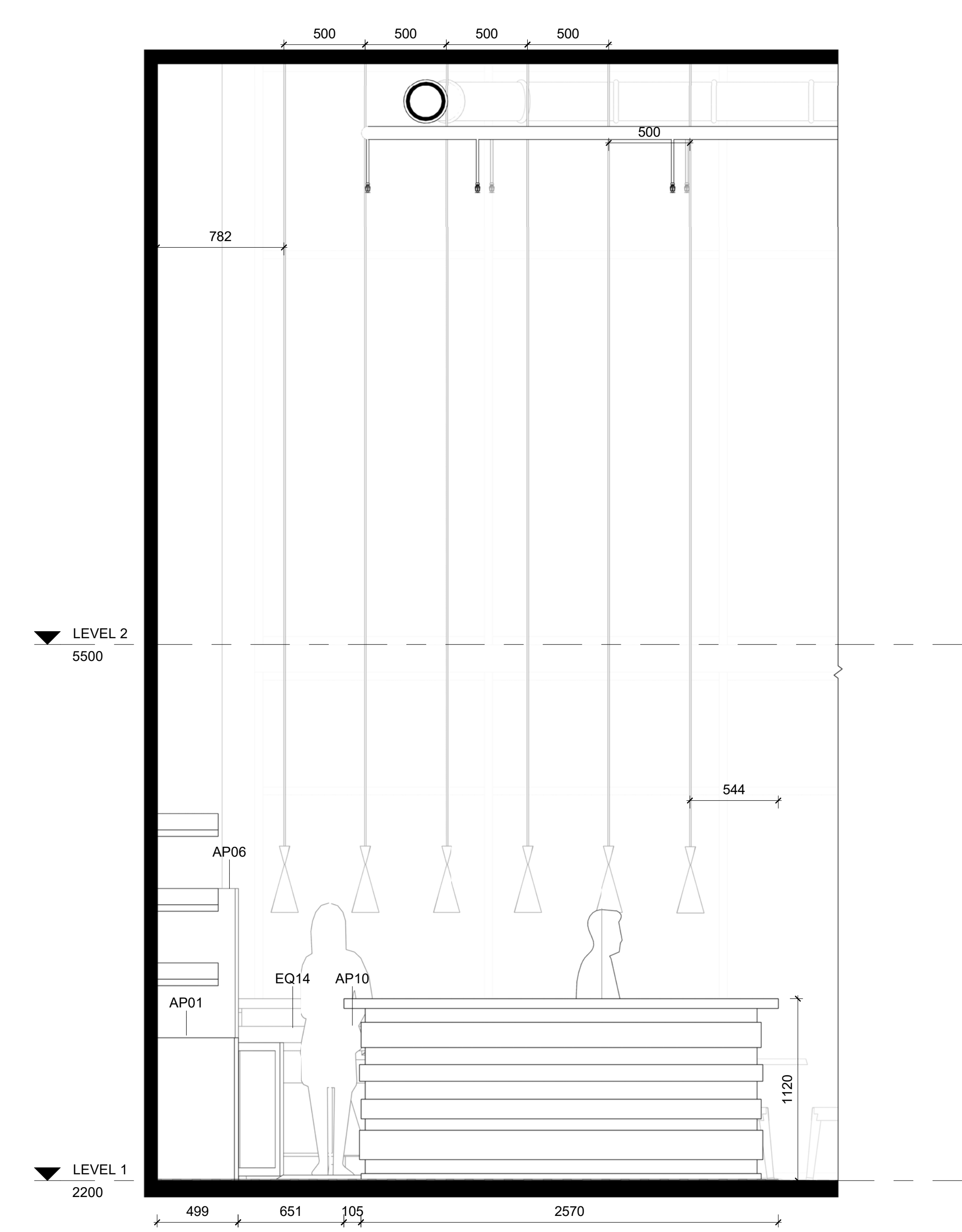
1 BAR Elevation 6 1 : 20
