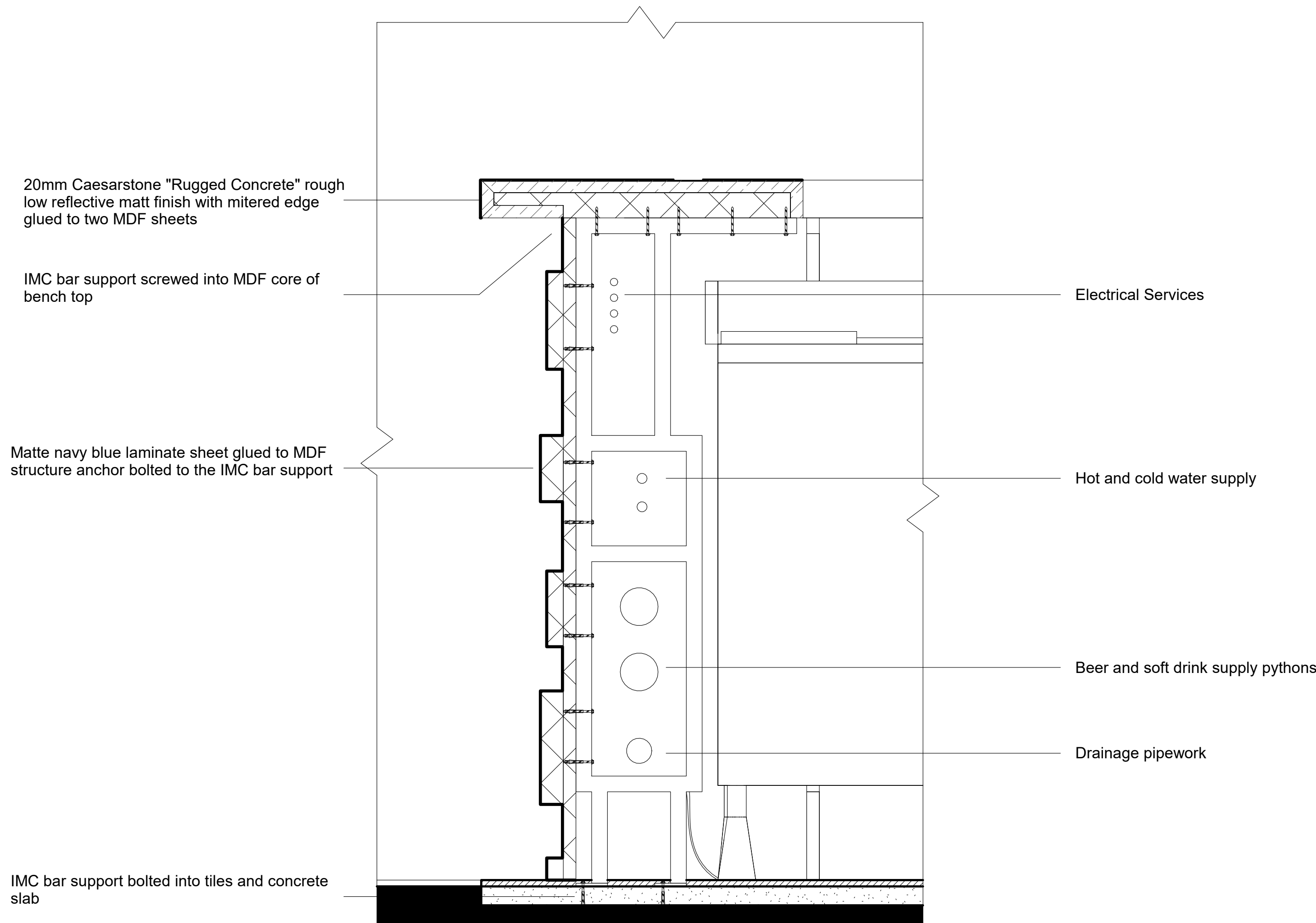
1 BAR Section - Bar 1 : 5
